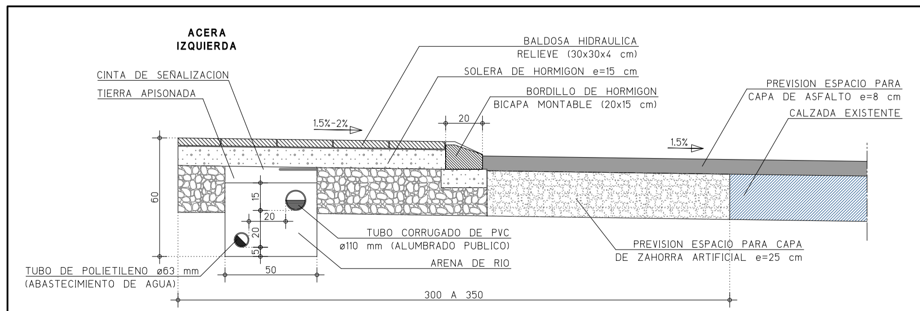
SECCION CONSTRUCTIVA CORRESPONDIENTE A LA SECCION A-A
