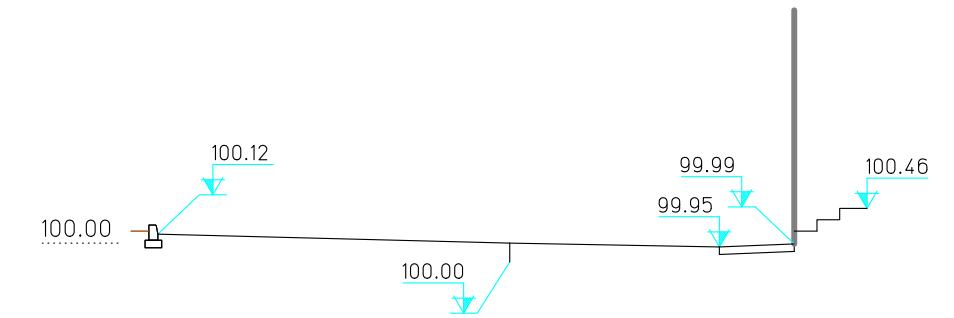
SECCION B-B E: 1/100
