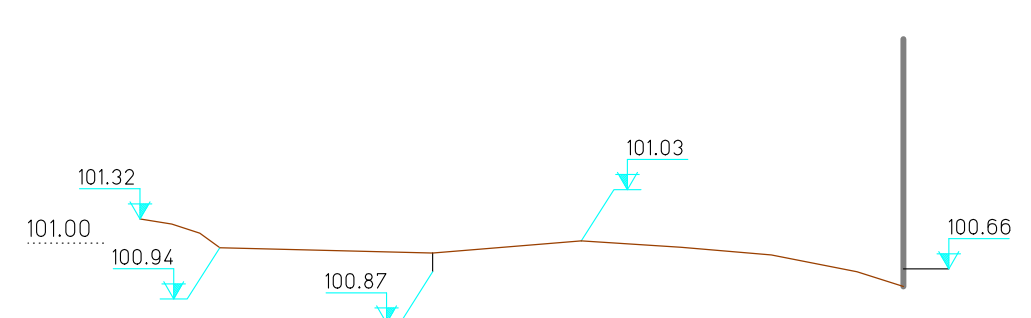
SECCION A-A E: 1/100
